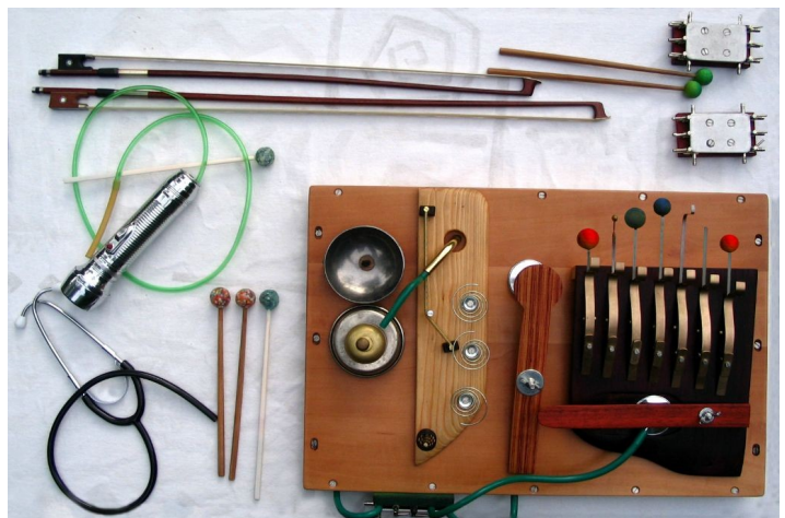
Musiscope 4 _ Musica
